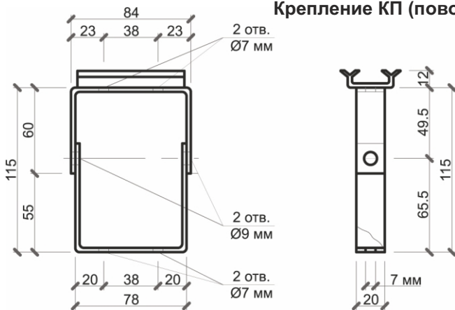
Крепление КП (поворотное)
