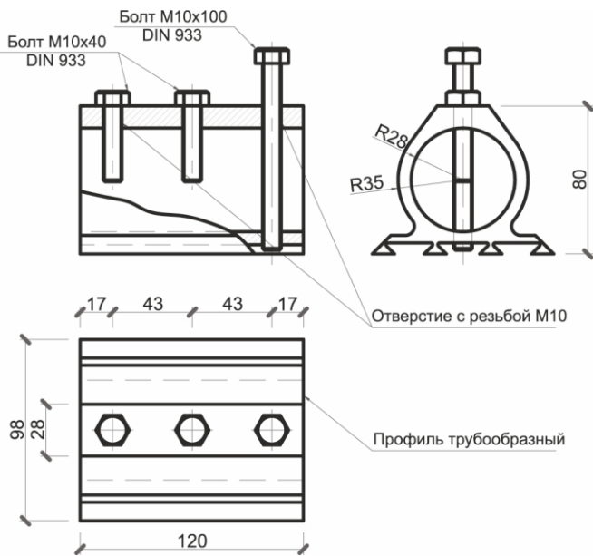
Крепление КП (поворотное)
