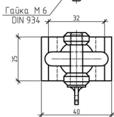
Крепление КПУ-25 (на трос)
