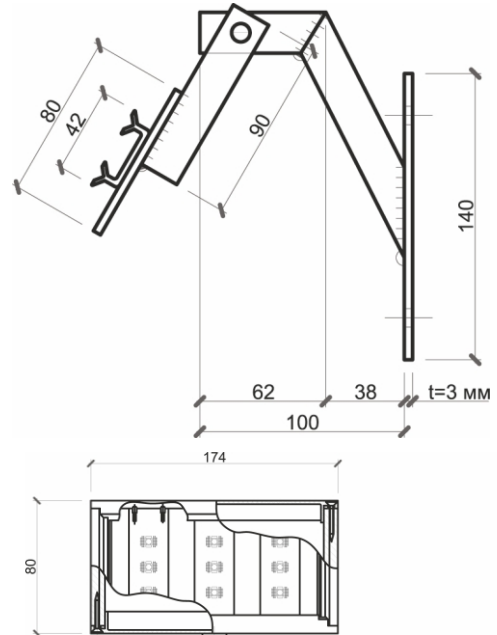
Крепление КПГ (поворотное)
