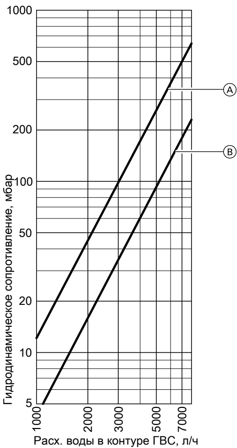
Гидродинамическое сопротивление контура ГВС
