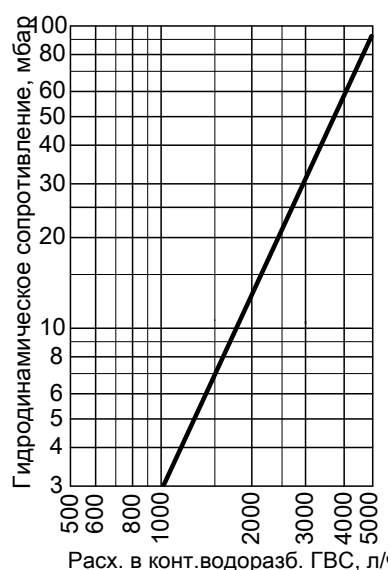
Производительность по горячей воде при номинальной тепловой мощности
