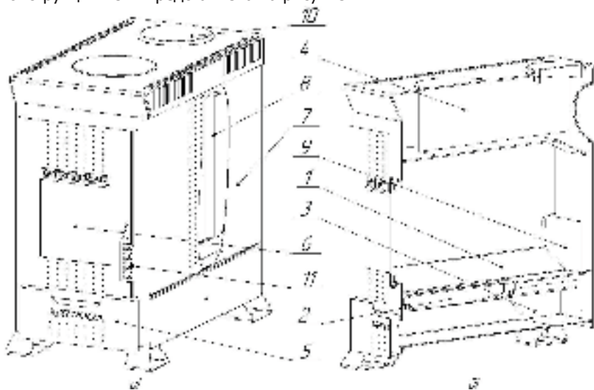
Рисунок 2 - Конструкция печи
