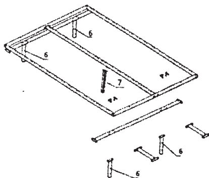
Рисунок 3. Установка ламелей
