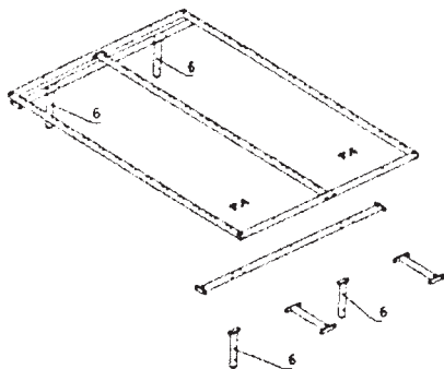
Рисунок 3. Установка ламелей
