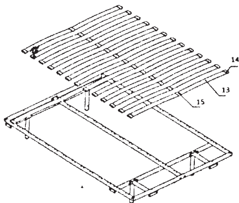
Рисунок 3. Установка ламелей
