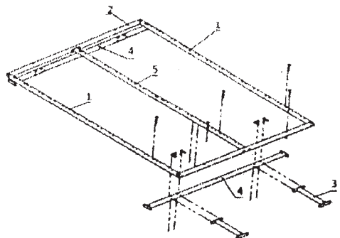
Рисунок 2. Установка ножек
