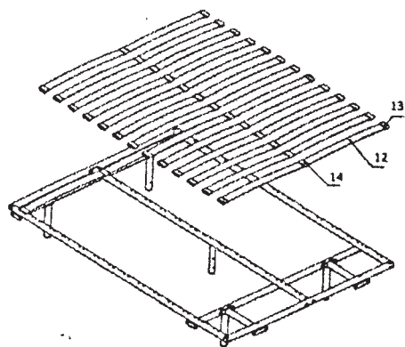
Рисунок 3. Установка ламелей
