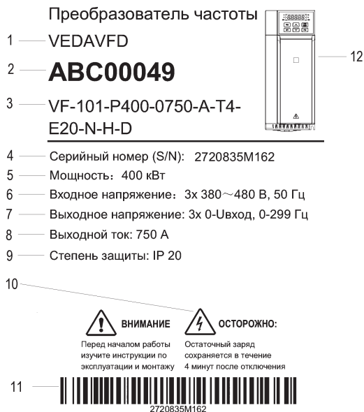
Рисунок 1.3-1. Пример маркировки преобразователя частоты
