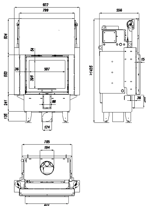
Rysunek 5. Rzuty z wymiarami wkładu kominkowego DEFRO HOME NAVI SM G.
