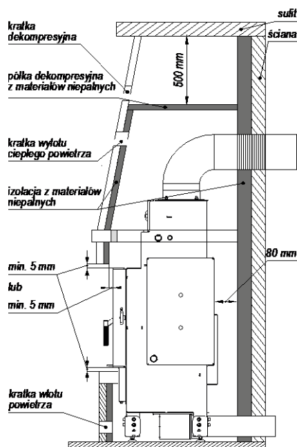
Rysunek 8. Przykładowa zabudowa wkładu kominkowego.
