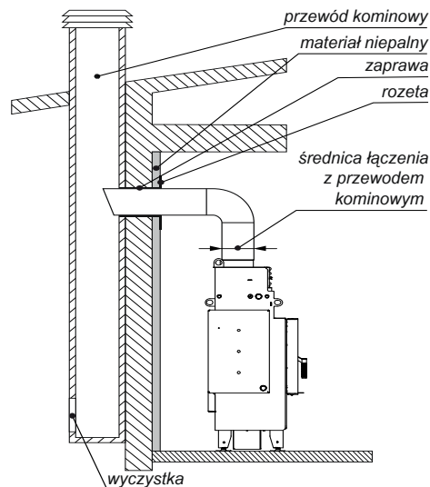
Rysunek 11. Podłączenie wkładu kominkowego do przewodu kominowego.
