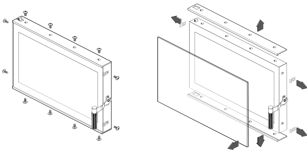
Rysunek 19. Demontaż szyby w drzwiach.
