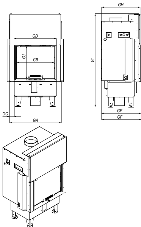
Rysunek 6. Rzuty z wymiarami wkładu kominkowego DEFRO HOME NAVI G w wersji z osłonami.
