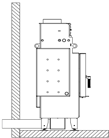
Rysunek 10. Podłączenie wkładu kominkowego do zewnętrznego wlotu powietrza.
