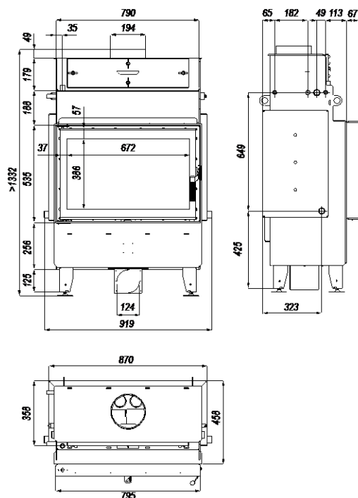
Rysunek 3. Rzuty z wymiarami wkładu kominkowego DEFRO HOME NAVI ME.
