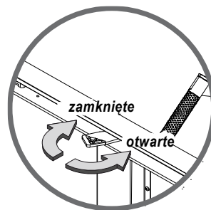
Rysunek 14. Ustawienie suwaka regulacji dopływu powietrza
