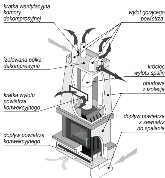
Rysunek 9. System dystrybucji gorącego powietrza.
