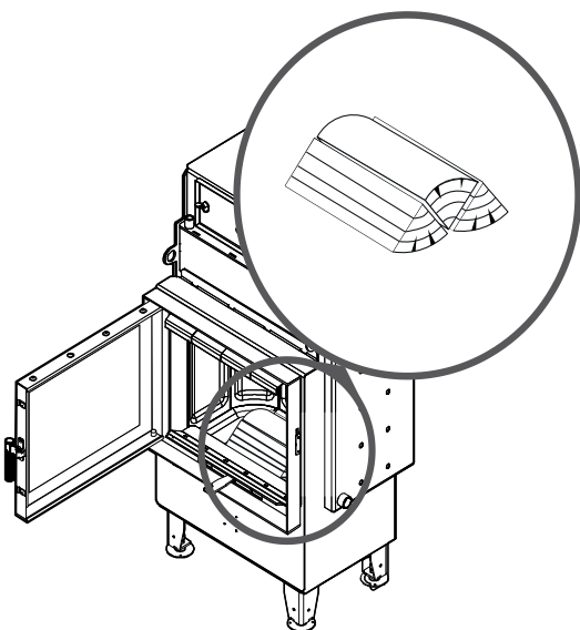
Rysunek 15. Sposób ułożenia paliwa
