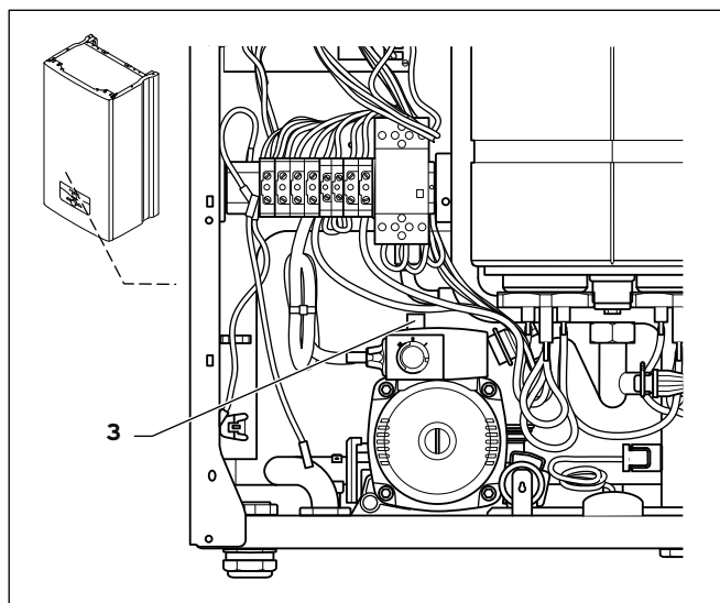
6.2 Brzi odzračnik
