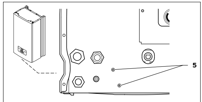
10.2 Крепежные винты на нижней стороне аппарата
