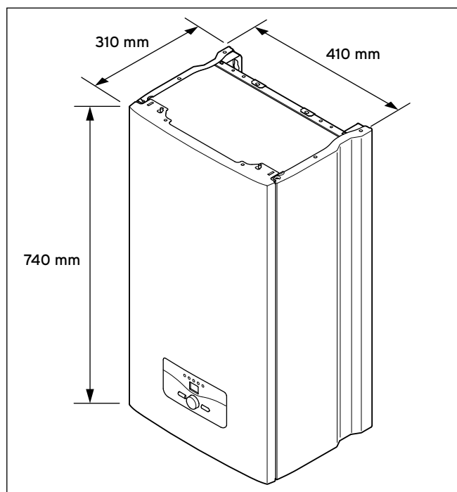
4.4 Priključne mjere u mm
