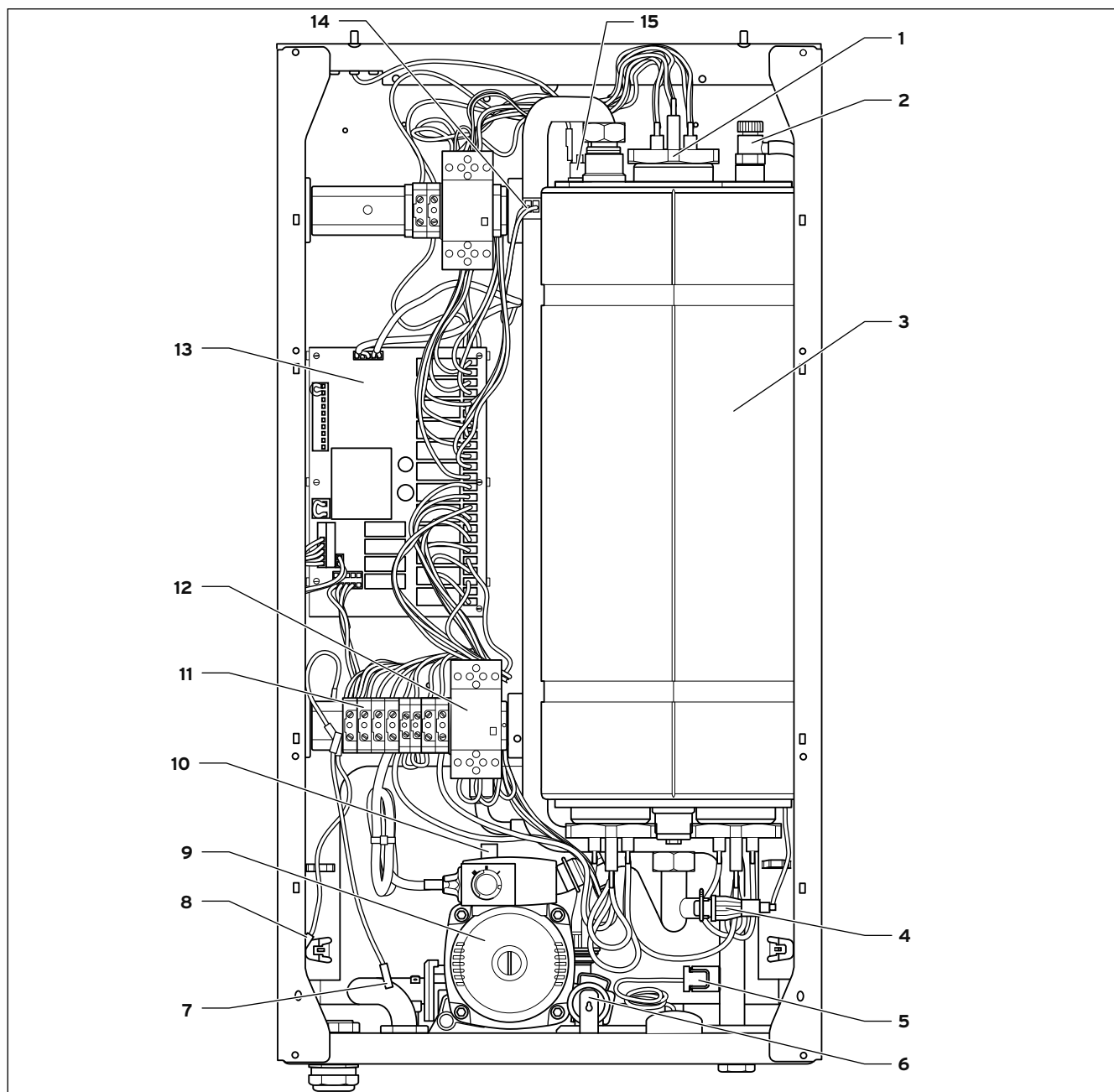
3.1 Вид спереди, аппарат открыт
