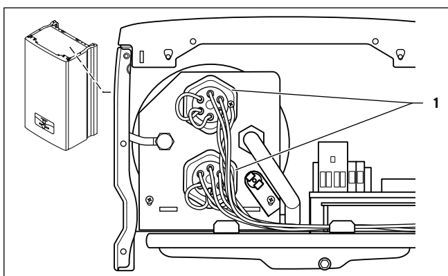
10.6 Демонтаж ТЭНа
