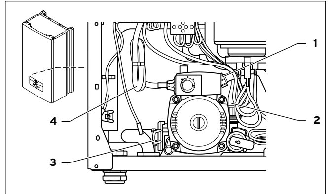
10.1 Демонтаж отопительного насоса
