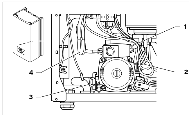
10.1 Izgradnja crpke
