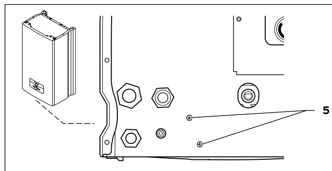
10.2 Vijci za pričvršćivanje na donjoj strani uređaja
