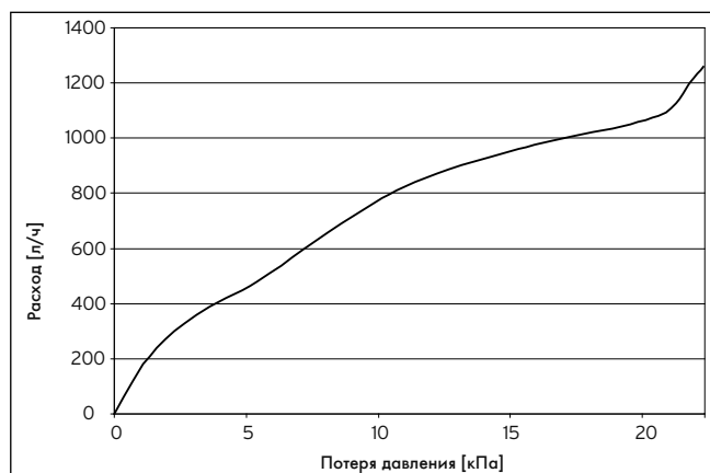
13.1 Потеря давления eIoBLOCK
