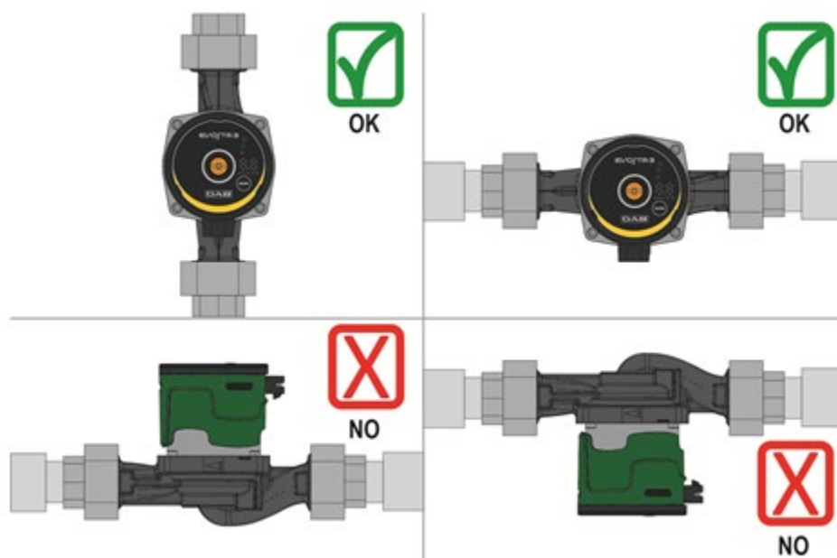
Рисунок 3: Монтажное положение
