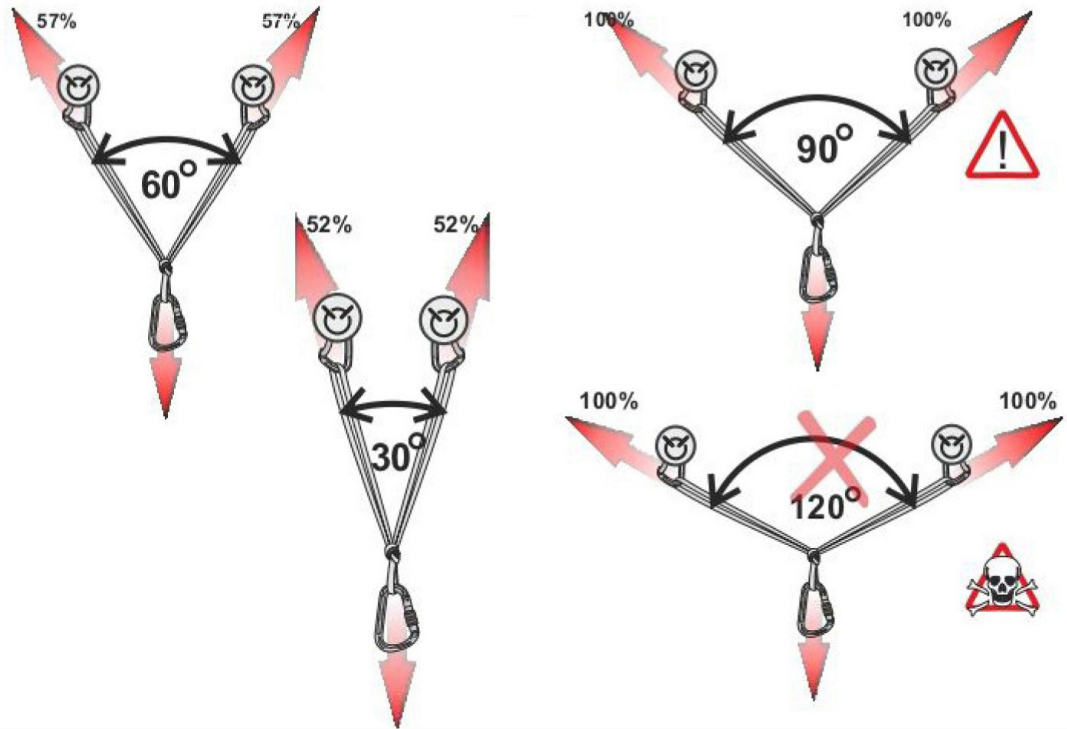
Рис. 3. Распределение нагрузок на анкерные точки в зависимости от углов
