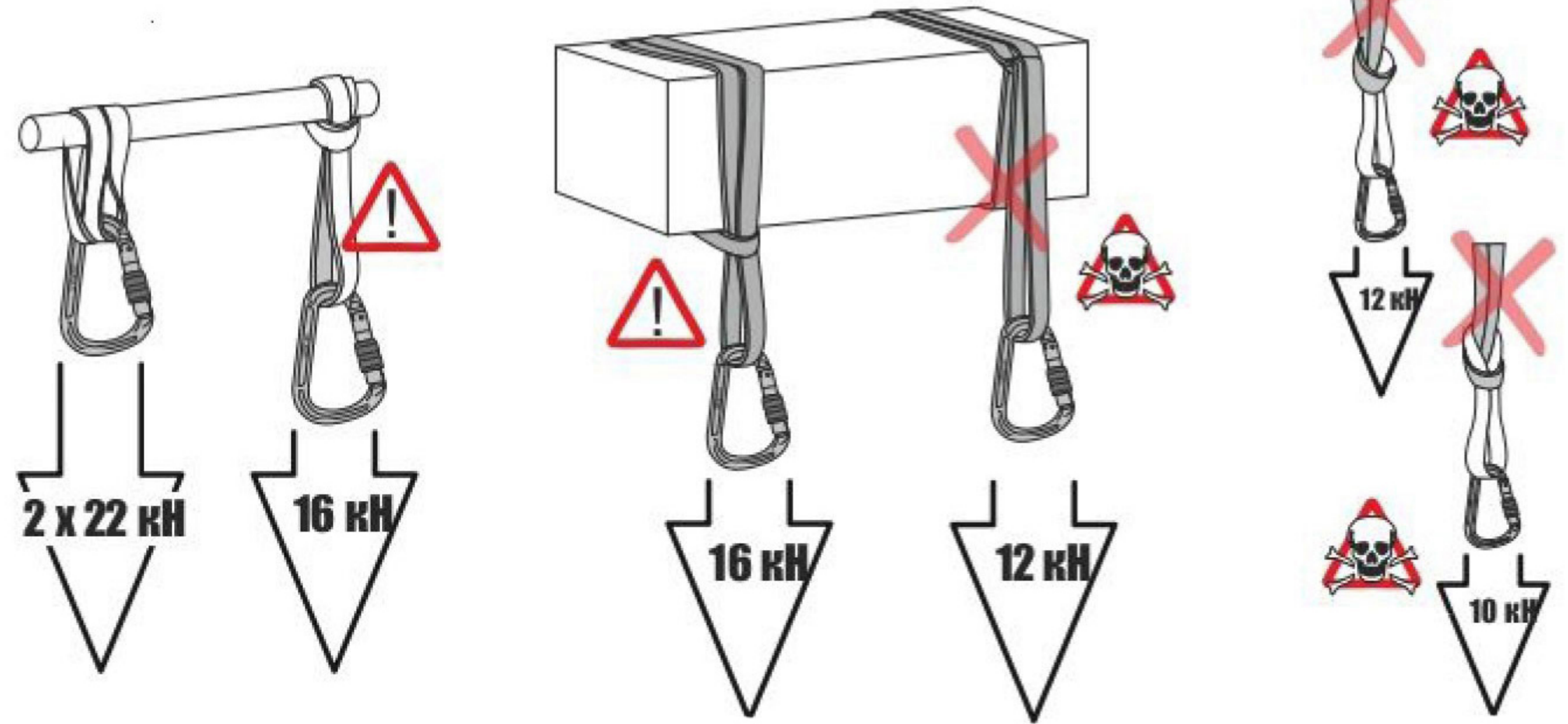
Рис. 2. Способы применения и выдерживаемые нагрузки
