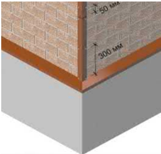
Рис. 16. Устройство внешних углов при помощи металлических уголков.
