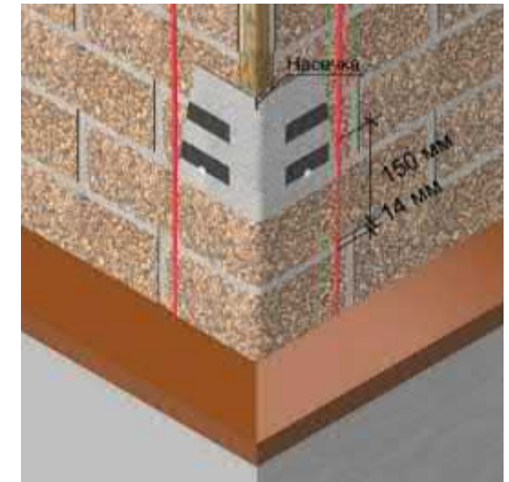
Рис. 21. Монтаж последующих угловых элементов.
