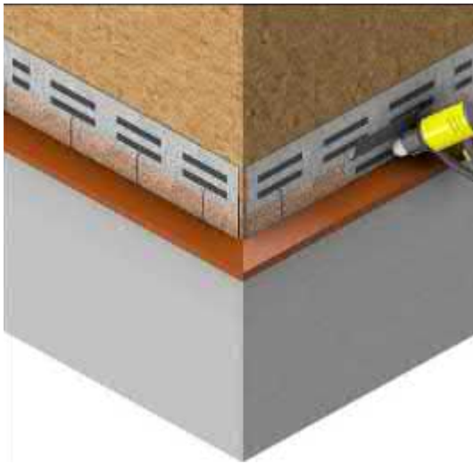
Рис. 15. Прогрев клеевых полос фасадной плитки строительным феном.
