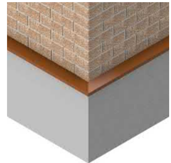
Рис. 22. Устройство внешних углов при помощи угловых элементов.
