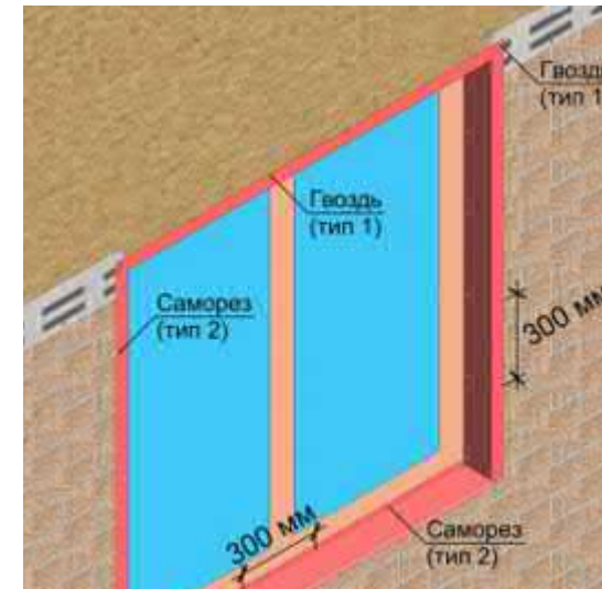
Рис. 27. Крепление металлических наличников.
