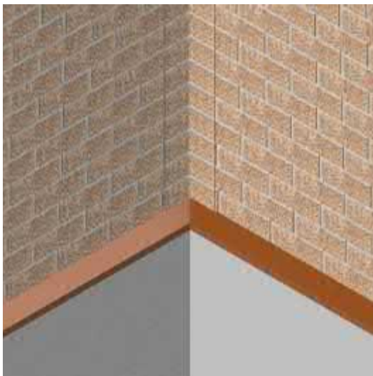
Рис. 24. Устройство внутренних углов при помощи угловых элементов.
