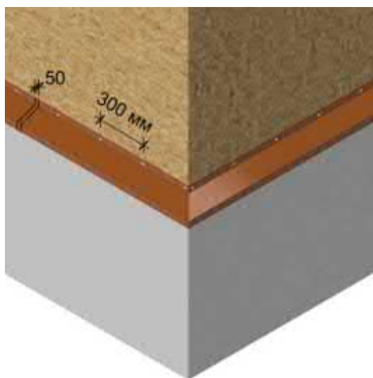
Рис. 6. Крепление металлических отливов.
