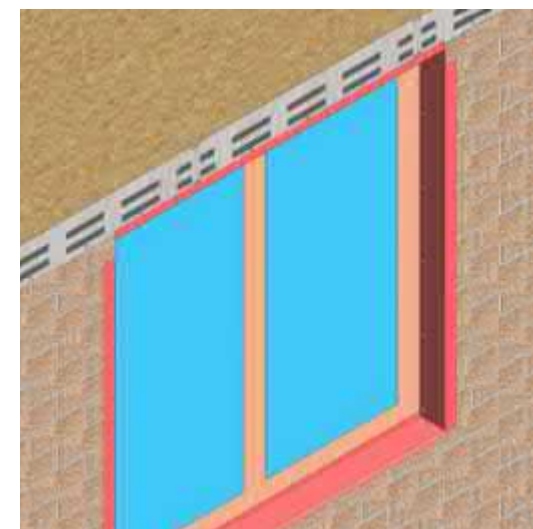
Рис. 28. Монтаж фасадной плитки над окном.
