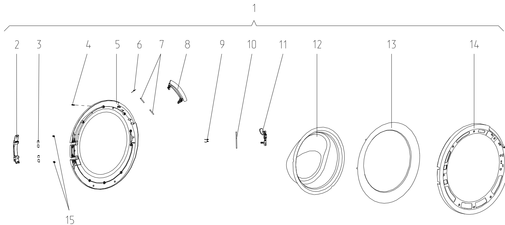
Рисунок 5 - Дверь
