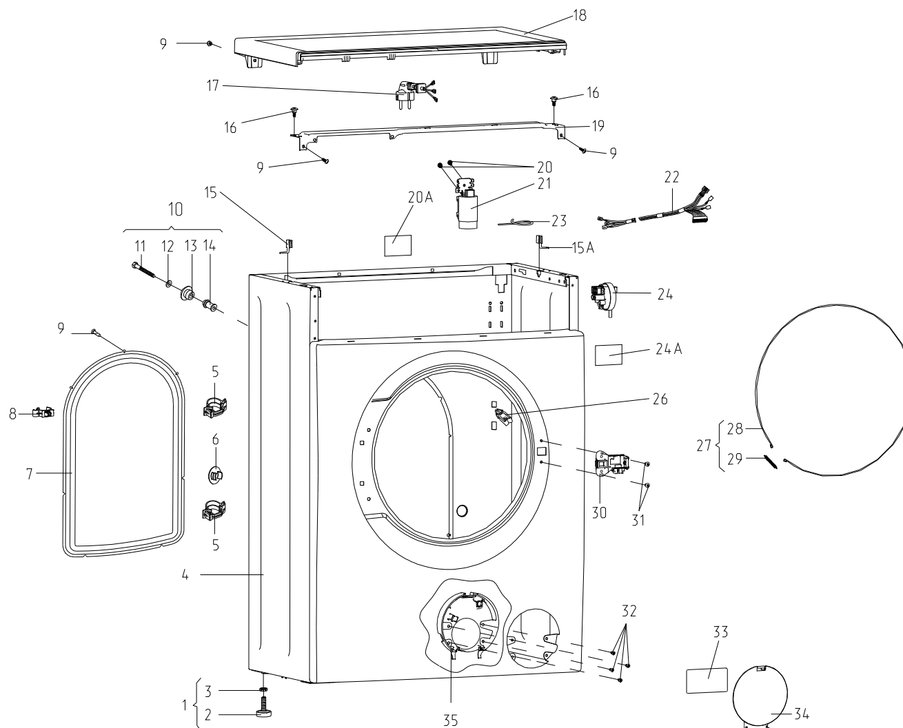
Рисунок 1 - Корпус
