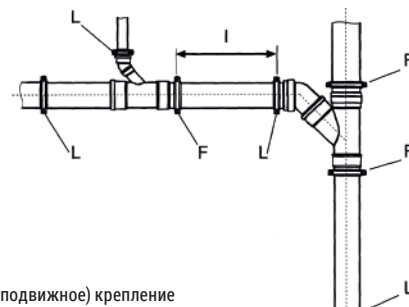
ХОМУТ С ПРОКЛАДКОЙ КАК ПЛАВАЮЩЕЕ КРЕПЛЕНИЕ
