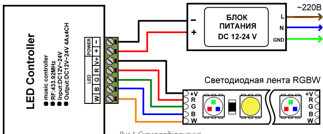
Рис.1. Схема подключения.
