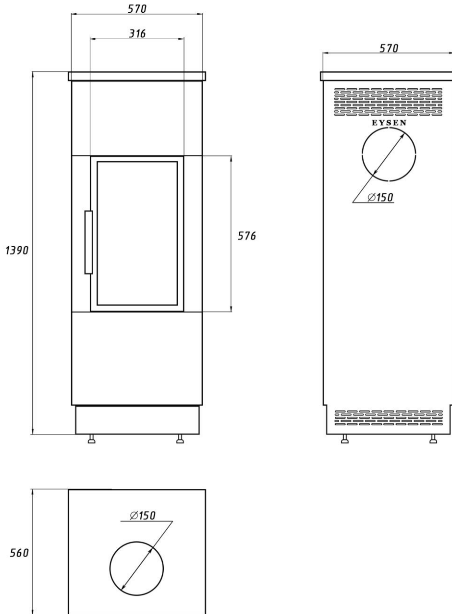
Схема печь-камин Tabaco Grey
