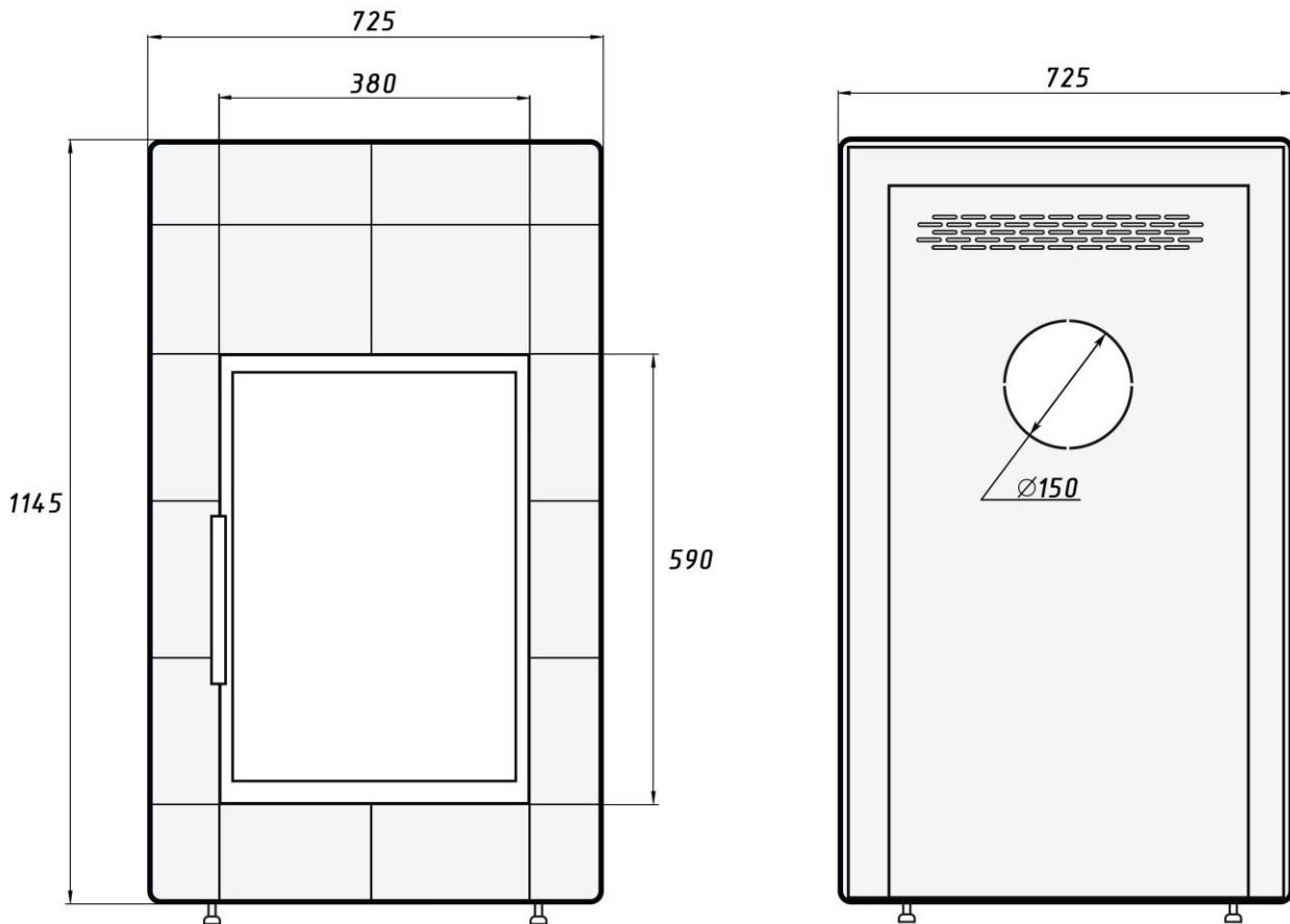
Схема печь-камин Atacama
