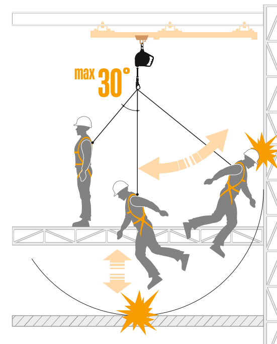
Рис. 5 Падение работника, сопровождающееся маятниковым движением.
