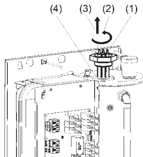
Рисунок 9. Замена блока ТЭН
