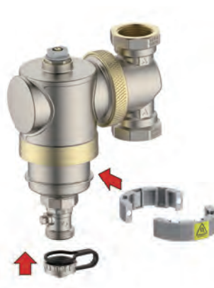
3. Закрыть дренажный клапан и надеть магнитный пояс
