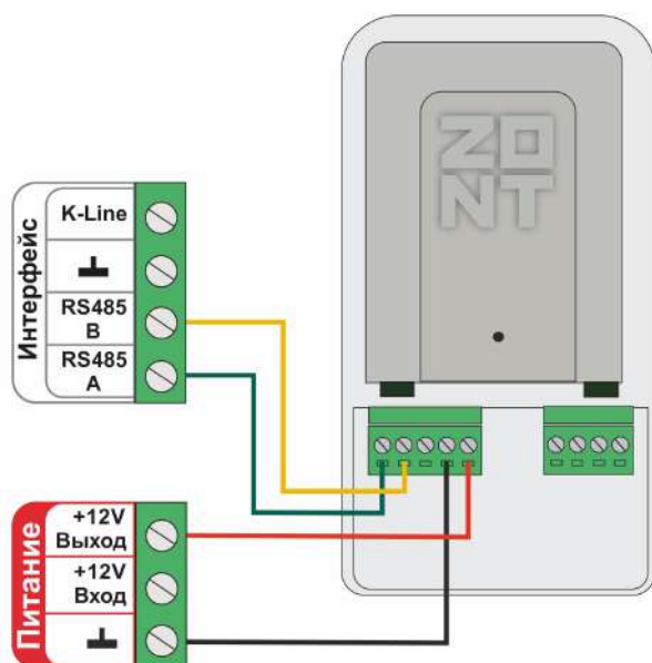
Схема подключения внешнего адаптера цифровой шины ECO по RS-485 :
