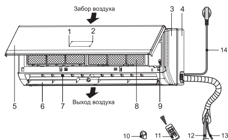
Внутренний блок
