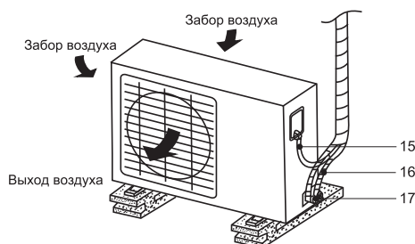
Наружный блок
