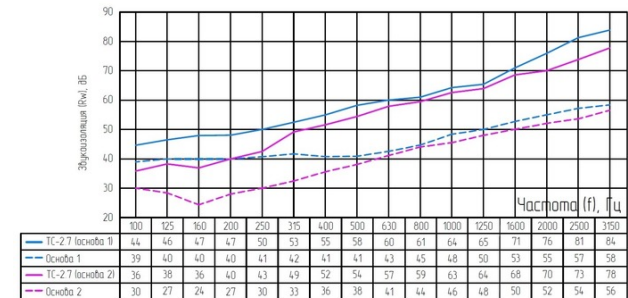
Частотные характеристики изоляции воздушного шума, R_w(f)
