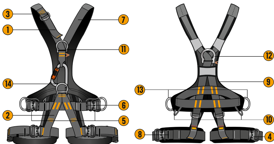
Рис. 1 Страховочная привязь PROMALP PRO, арт. HS-73C.
