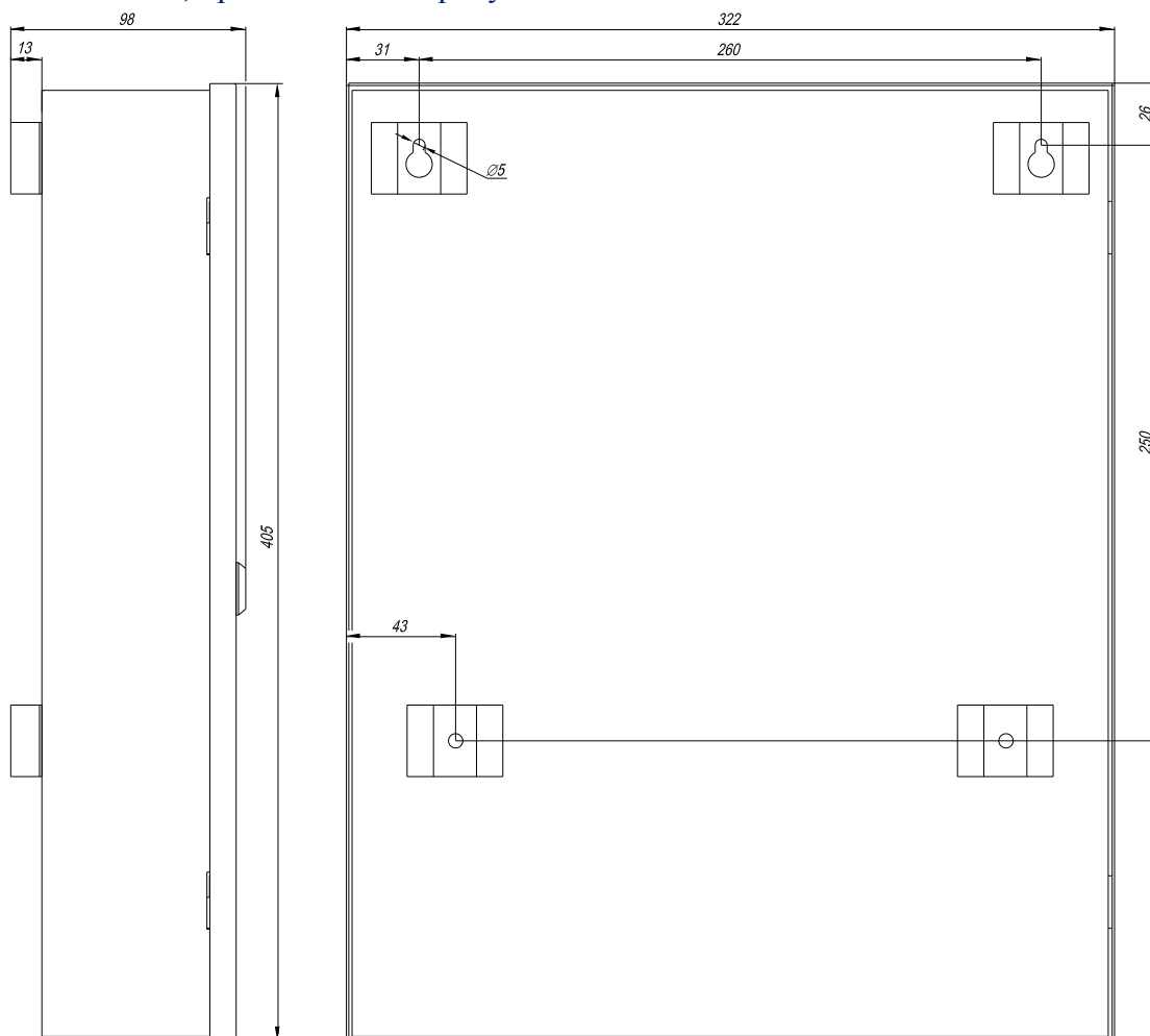
Рис. 61. Установочный чертеж основания корпуса ППКО серии «А24М»
