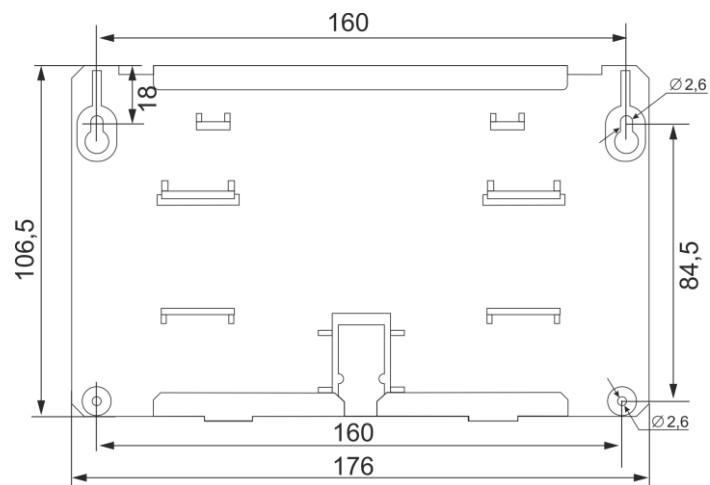
Рис. 63. Установочный чертеж основания корпуса P485
