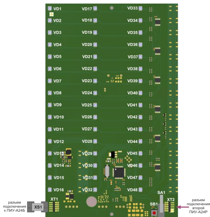
Рис. 51. Внешний вид платы ПИУ-А24Р(О), обозначение элементов и схема подключения Назначение элементов и контактов на плате ПИУ-А24Р(О) приведено в таблице 32.
