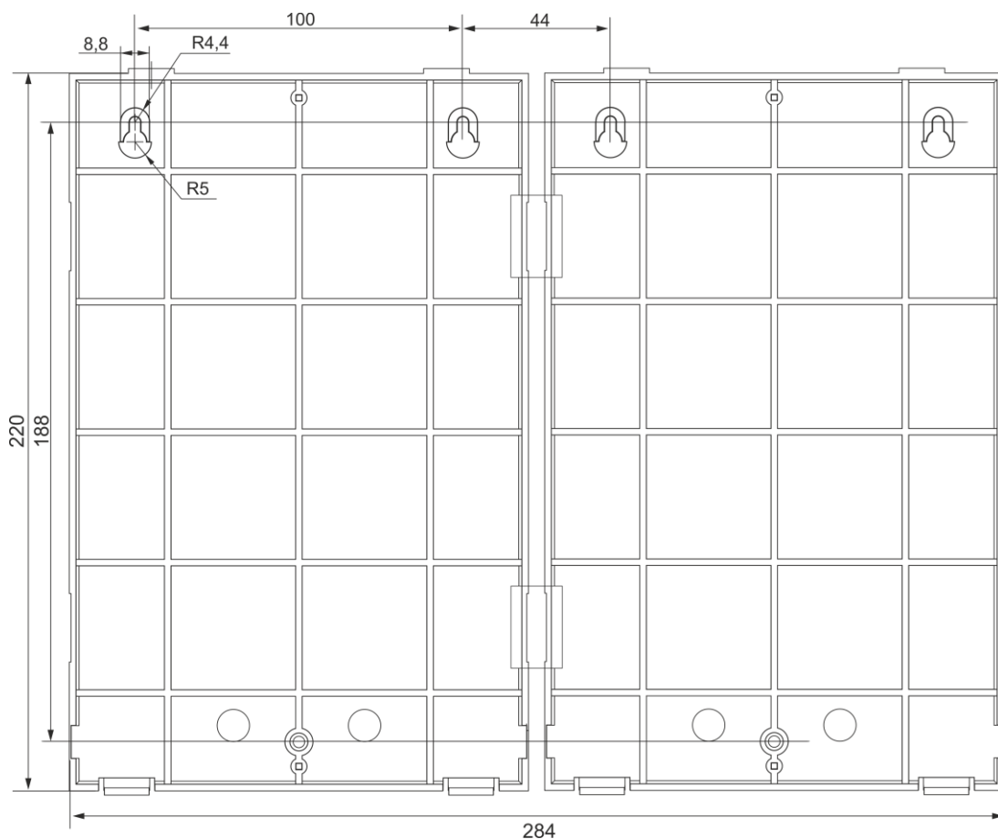
Рис. 65. Установочный чертеж ПИУ-А24Б(О) с одной подключенной ПИУ-А24Р(О)
