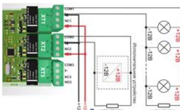
Рис. 6. Внешний вид и обозначение элементов РМ-А24/3
