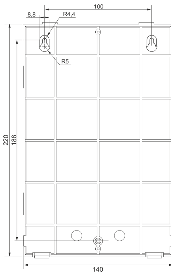
Рис. 64. Установочный чертеж ПИУ-A24Б(O)
