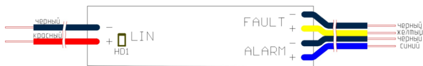
Рис. 55. Внешний вид МА-ХР777
