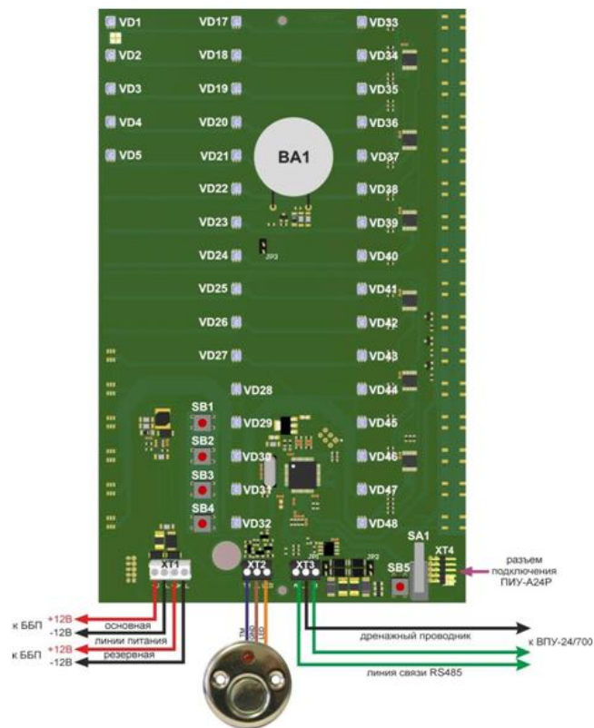
Рис. 48. Внешний вид и подключение платы ПИУ-A24Б(O)
