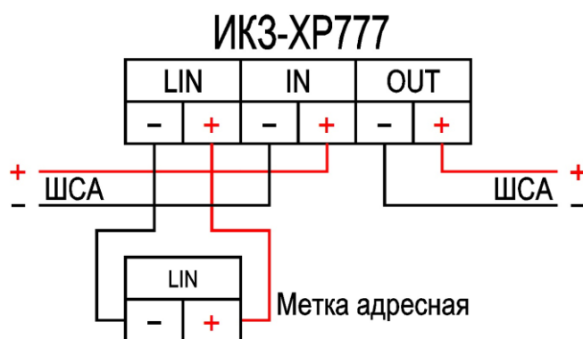
Рис. 60. Схема подключения изолятора
