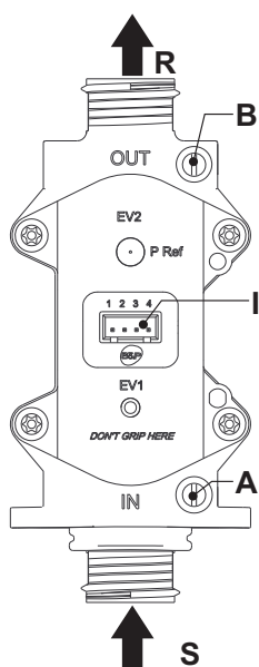
Рис. 29 - Газовый клапан
