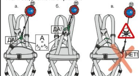
Рис. 4. Соединение НВ с привязью
