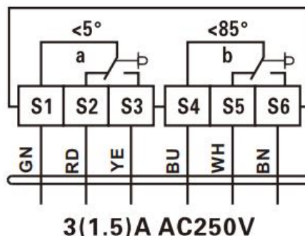
Концевые выключатели
