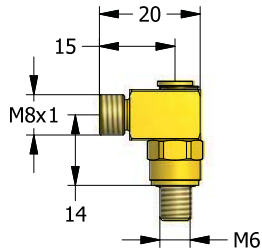
CF090 Угловой адаптер порта Winkelstück Elleboog-poortadapter Adaptateur de port coudé
