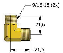
HTH90 Проходной угольник Winkelstück Bochtverbindingsstuk Raccord coudé
