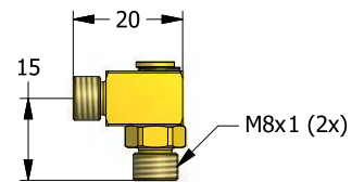
CTH90 Угловое соединение Winkelstück Bochtverbindungsstuk Raccord coudé
