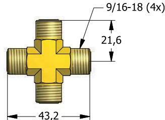
HTH94 Проходная крестовина Kreuzstück Verbindingskruisstuk Raccord croisé
