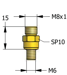
CF111 Адаптер порта Anschlussadapter Poortadapter Adaptateur de port
