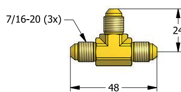
VTH93 Соединительный тройник Anschlussmuffe T-stuk Raccord en T
