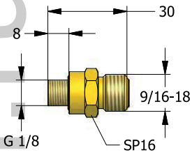
GF118 Адаптер порта Anschlussadapter Poortadapter Adaptateur de port
