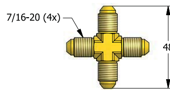
VTH94 Проходная крестовина Kreuzstück Verbindingskruisstuk Raccord croisé
