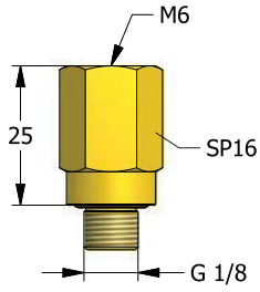
CF118 (G 1/8) Адаптер порта Anschlussadapter Poortadapter Adaptateur de port
