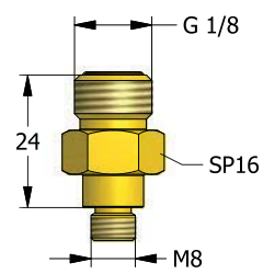
CF188 (G 1/8 - M8) Соединение Anschluss Koppeling Raccord
