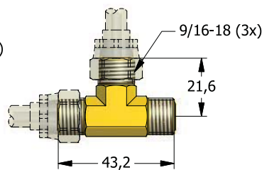
HTH93 Соединительный тройник Anschlussmuffe T-stuk Raccord en T
