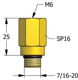
CF716 (7/16) Адаптер порта Anschlussadapter Poortadapter Adaptateur de port
