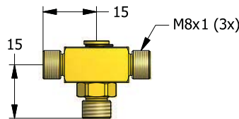
CTH93 Тройное соединение Anschlussmuffe T-stuk Raccord en T
