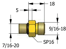
CF118 Адаптер порта Anschlussadapter Poortadapter Adaptateur de port
