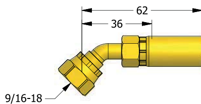
HF145 муфта 45° 45° Drehgelenk 45° scharnier 45° basculement
