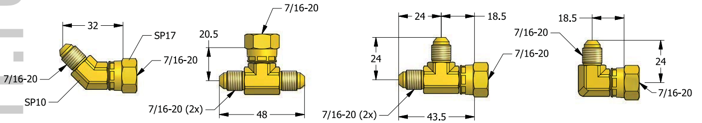
VS090 Угловой фитинг 45° с накидной гайкой 45° Überwurfmutter winkelstück Wartelmoer elleboogstuk 45° Écrou-chapeau coudé 45°
