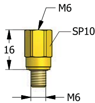
CF110 Удлинитель адаптера порта Verlängerungsadapter Uitbreiding poortadapter Rallonge adaptateur de port
