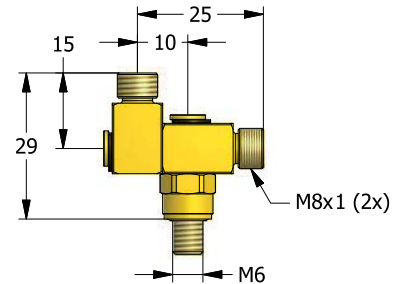
CF093 Адаптер порта - тройник с боковым отводом T-muffe anschlussadapter Loop poortadapter aftakking Adaptateur de port en T
