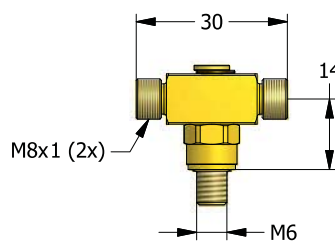
CF094 Тройниковый адаптер порта Abzweigmuffe anschlussadapter Poortadapter aftakking Adaptateur de port en T
