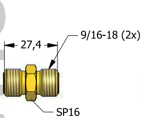
HTH10 Соединение Anschluss Koppeling Raccord
