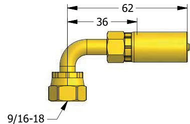
HF190 муфта 90° 90° Drehgelenk 90° scharnier 90° basculement
