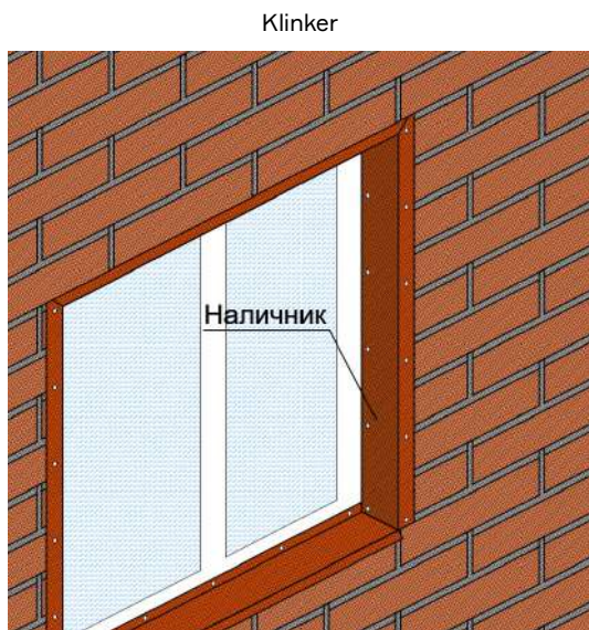
Рис. 29. Внешний вид оконного проёма с наличником с посыпкой (тип 4, таблица №2).
