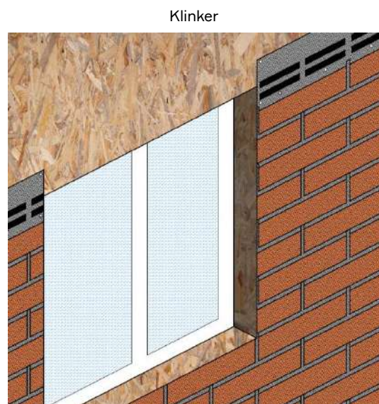
Рис. 26. Монтаж фасадной плитки вокруг оконного проёма.
