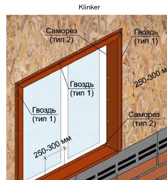
Рис. 31. Обрамление оконного проёма при помощи наличника 3D (тип 5, таблица №2).
