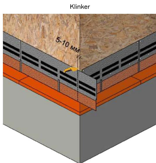
Рис. 14. Подрезка фасадной плитки при подходе к углам.
