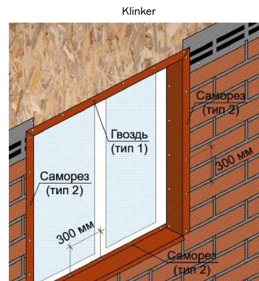
Рис. 27. Крепление металлических наличников с посыпкой.
