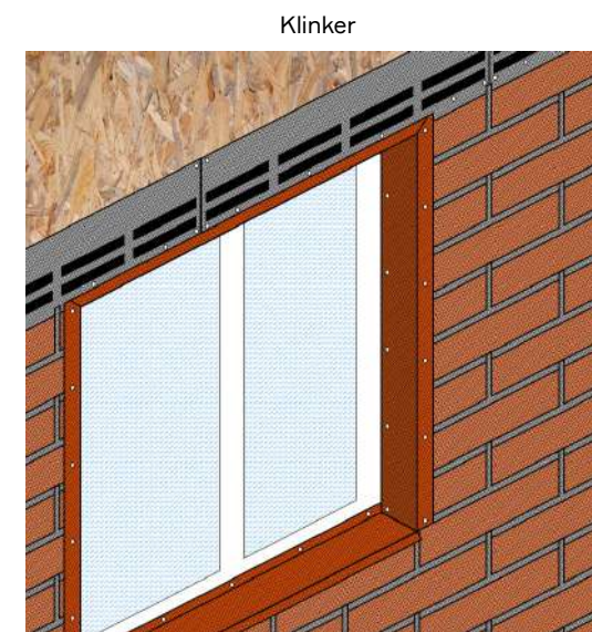
Рис. 28. Монтаж фасадной плитки над оконным проёмом.
