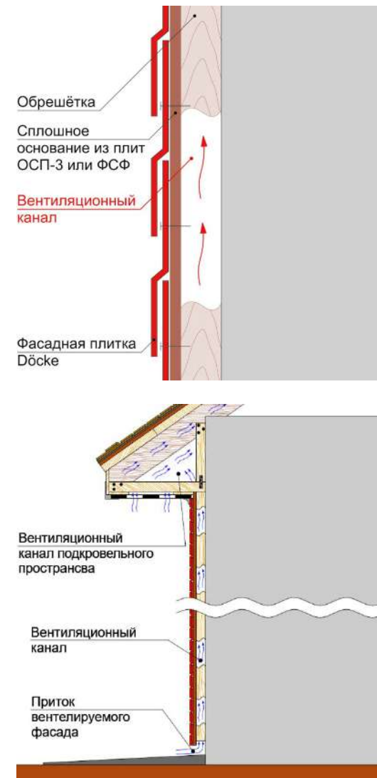
Рис. 1. Схема вентилируемого фасада на примере фасадной плитки Döcke.
