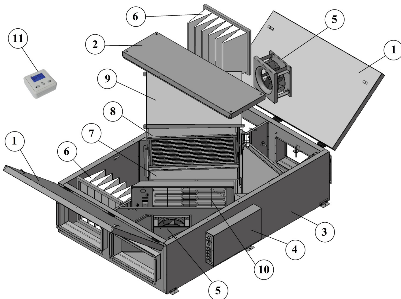
Состав установок
