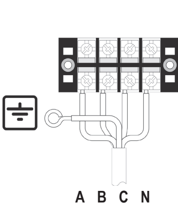
Рис. 3. Схема 3-фазного подключения электрокотла
