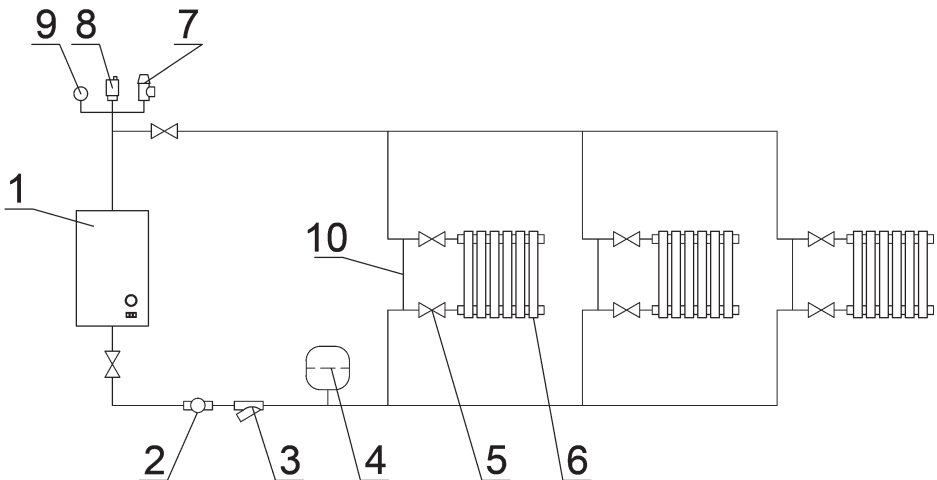
Рис. 5. Упрощённая схема подключения электроротла в закрытую отопительную систему с циркуляционным насосом.
