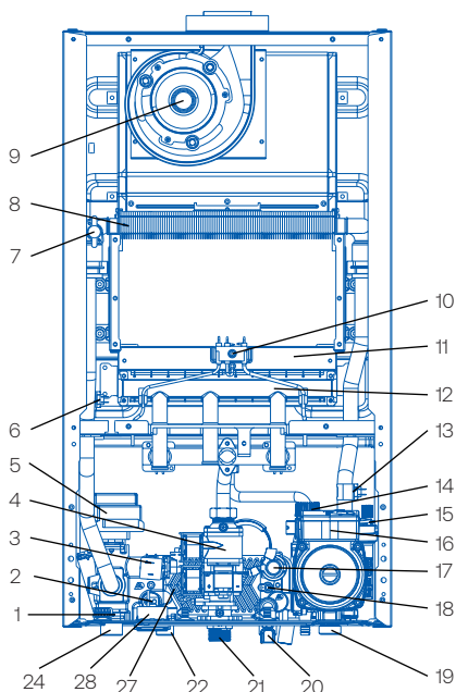
Двухконтурные котлы: TechLine S 2.10/2.14/2.18/2.24/2.28TW(TWs)
