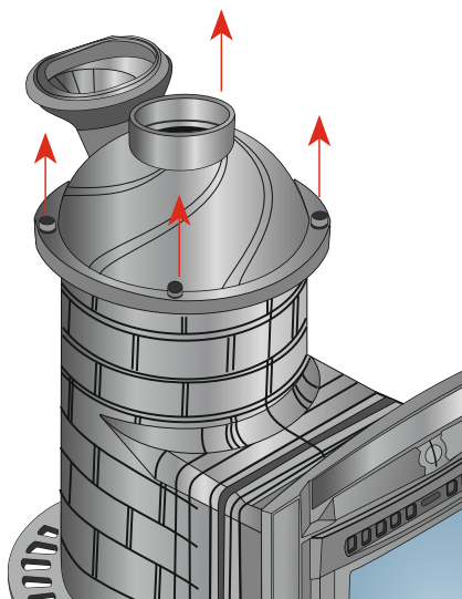
а) Откручиваем 4 болта крепления купола.
