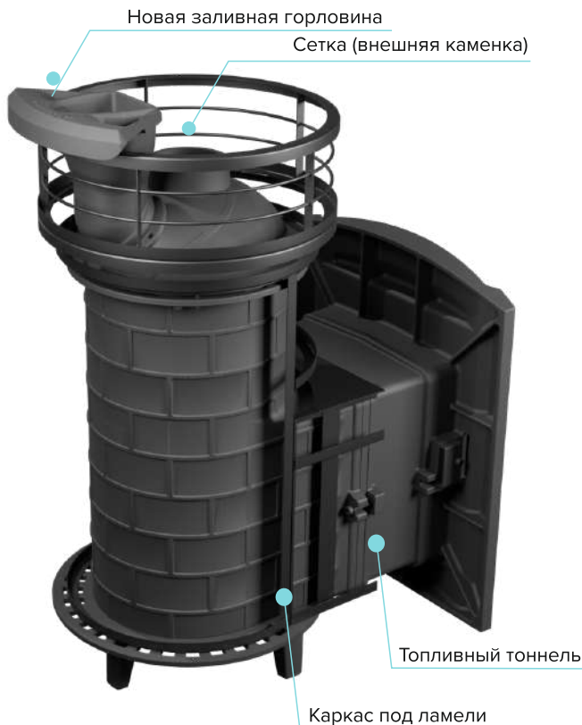
печь с закрытым (в облицовке) топливным тоннелем
