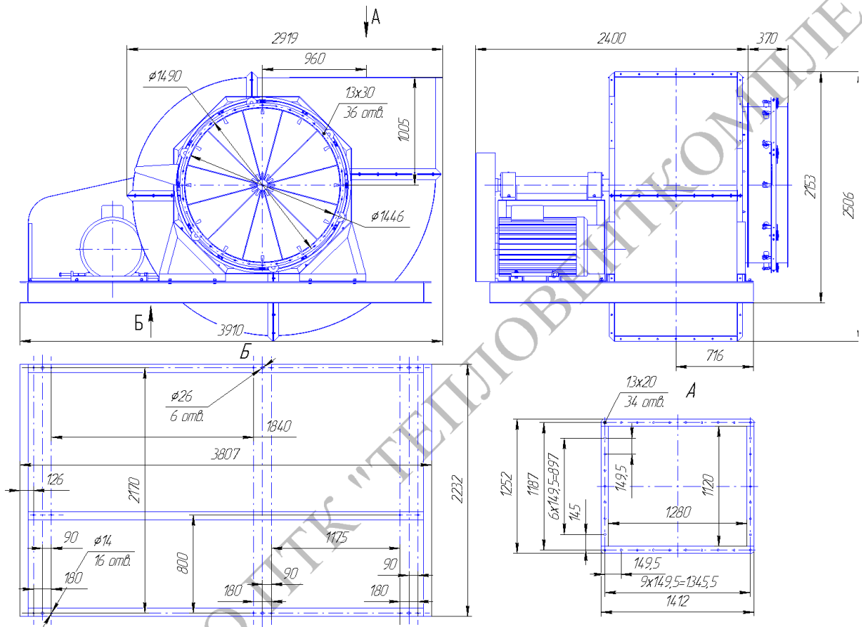
Вентилятор ВР 80-75 №16 исполнение 5-01. Габаритные и присоединительные размеры.
