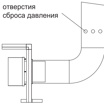
Рис. 9. Установка трубы дымоудаления
