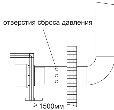
Рис. 10. Установка трубы дымоудаления
