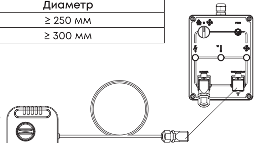
Рис. 11. Подключение внешнего температурного контроллера
