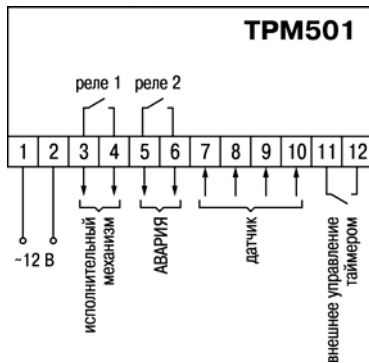
Рисунок Б.1 – Клеммник ТРМ 501
