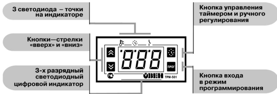
Рисунок 3.1 – Лицевая панель прибора
