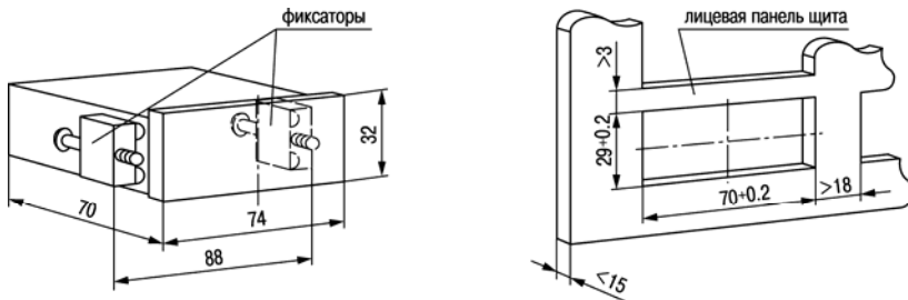
Рисунок А.1 – Габаритные и установочные размеры TRM501
