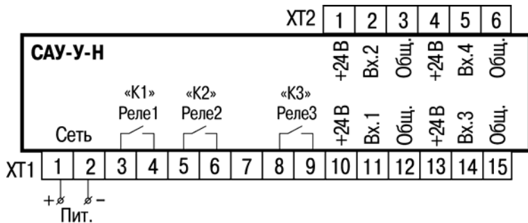
Рисунок Б.1 – Схема подключения САУ-У-Н
