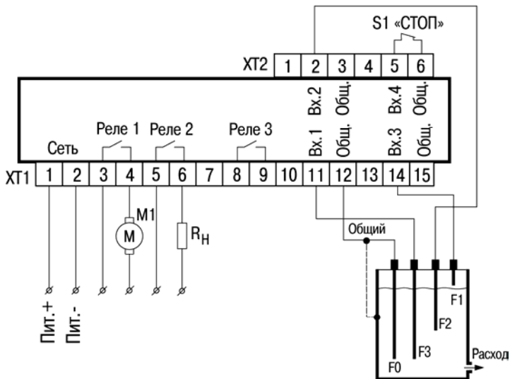
Рисунок В.1 – Схема подключения САУ-У-Н для выполнения алгоритма 01 M1 – исполнительное устройство (насос, электромотор, клапан или др.); R н – сигнализатор (звонок, сирена, лампа или блокирующий контактор); F1–F3 – кондуктометрические датчики уровня
