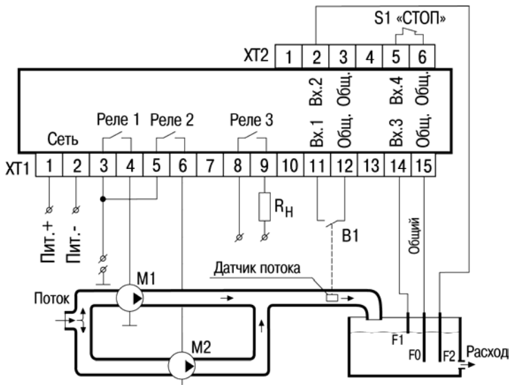
Рисунок В.8 – Схема подключения САУ-У-Н для выполнения алгоритма 12 M1 и M2 – насосы; R н – сигнализатор аварии или дополнительный насос; B1 – датчик потока; F1, F2 – кондуктометрические датчики уровня
