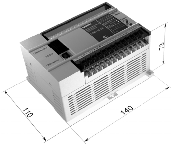
Рисунок А.2 – Габаритные размеры ПЛК110.X.32.X-X и ПЛК110.X.30.X-X
