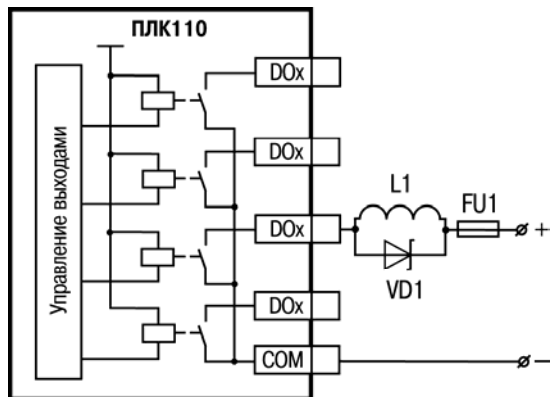
Рисунок В.7 – Подключение цепей защиты при реактивной нагрузке
