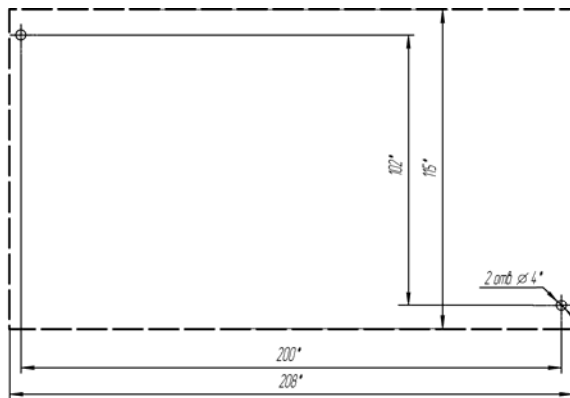
б) ПЛК110.X.60.X-X
