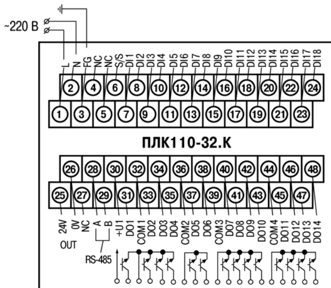
Рисунок Б.4 – Схема расположения и назначение клемм на ПЛК110-220.32.К
