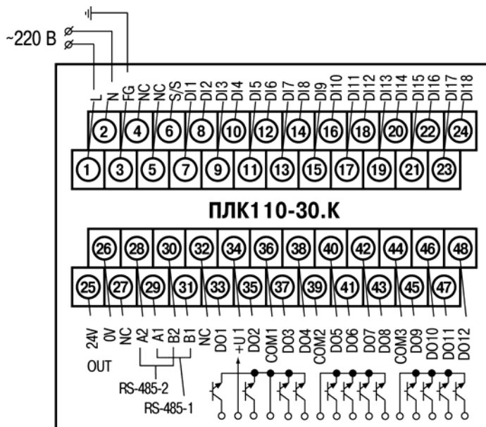
Рисунок Б.6 – Схема расположения и назначение клемм на ПЛК110-220.30.К
