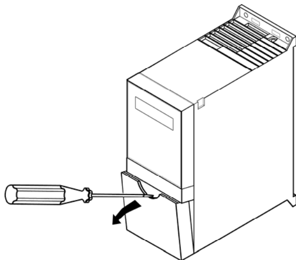
Рисунок 5.3 – Лицевая панель прибора. Клеммный отсек. Снятие крышки отсека
