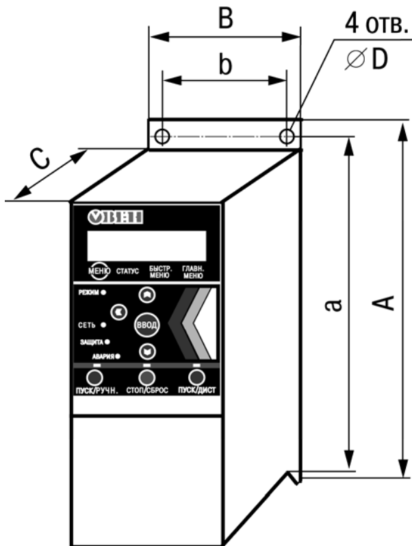
Рисунок А.1 - Габаритные и присоединительные размеры прибора модификаций 01 – 08 (расшифровка обозначений приведена в таблице А.1).
