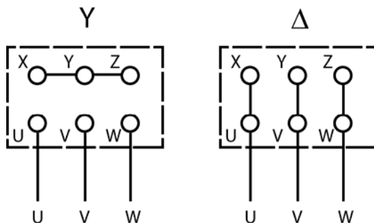
Рисунок 5.2 – Соединения по схемам «звезда» (слева) и «треугольник» (справа)
