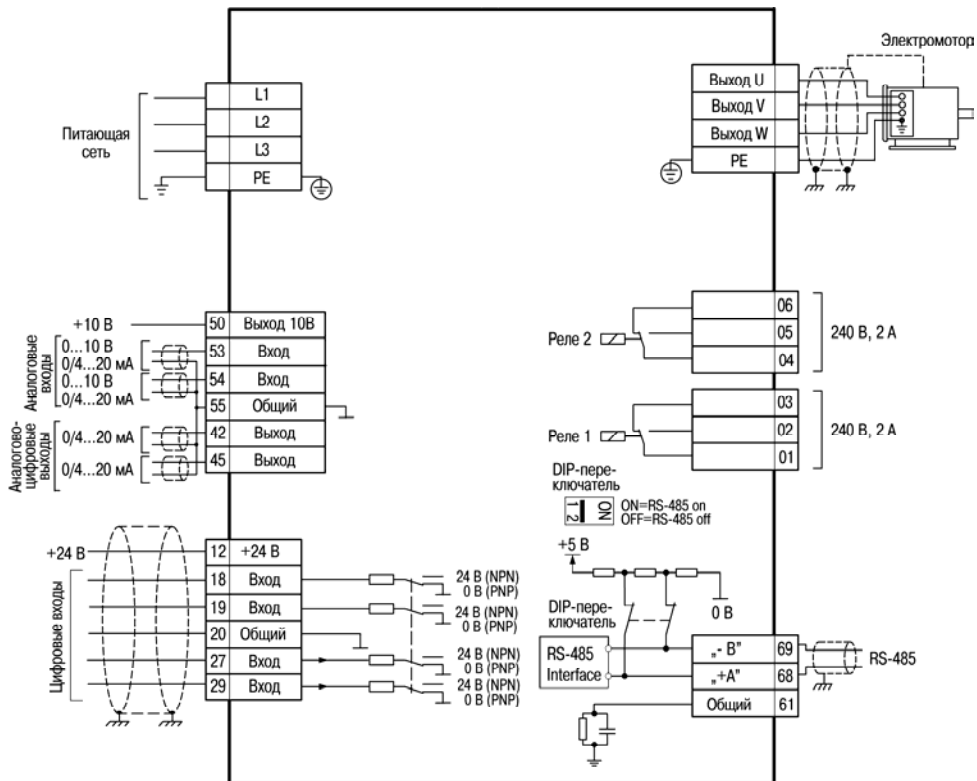
Рисунок Б.1 – Схема электрических соединений всех клемм прибора
