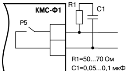
Рисунок 3.5 – Шунтирование контактов реле при работе с индивидуальными нагрузками
