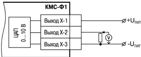
Рисунок 3.11 – Пример подключения выходного устройства типа «У»
