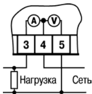
Рисунок Б.2 – Подключение прибора к однофазной сети
