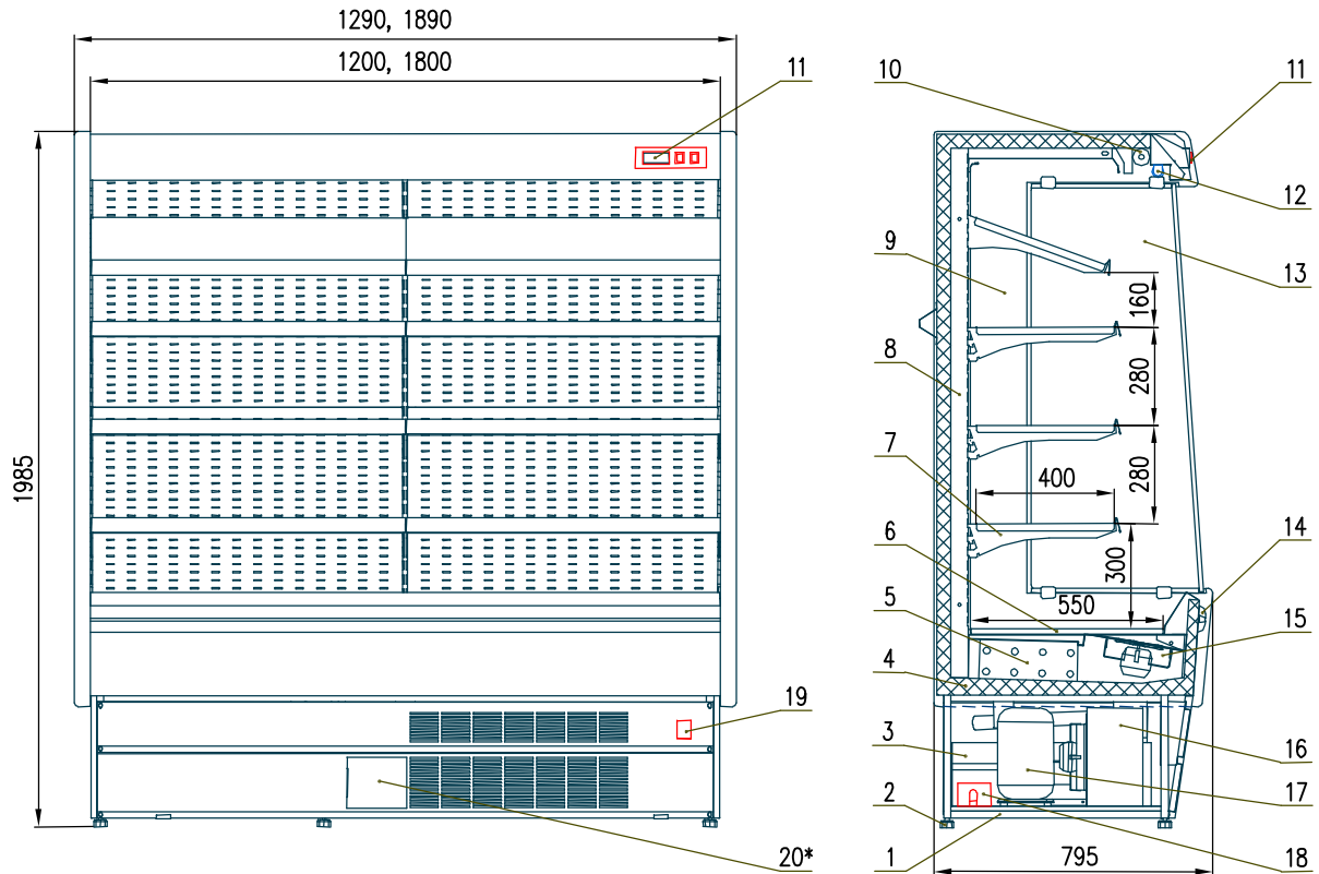
Рис. 1. Схема витрины «ВИЛИЯ» П ВСН:
