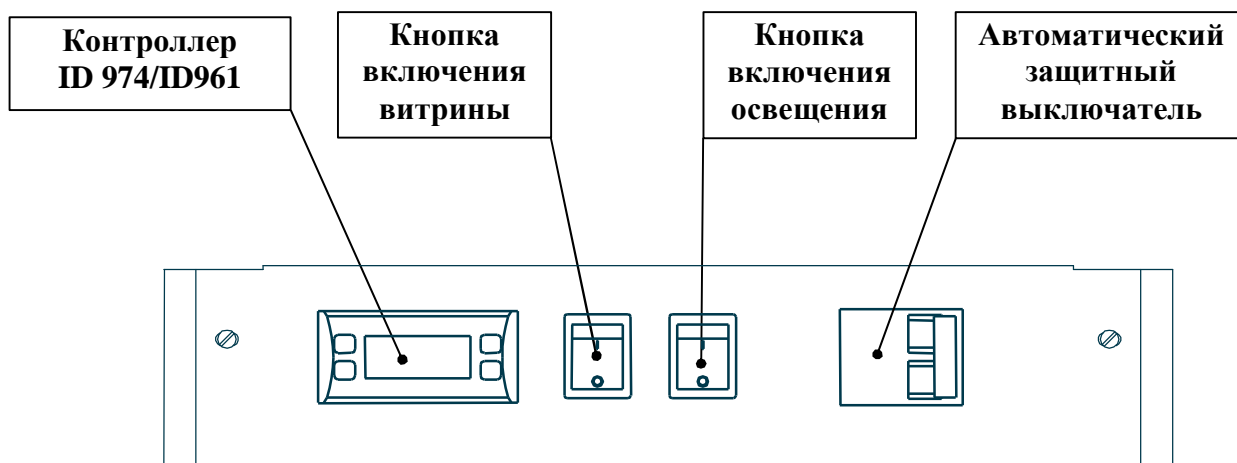
Рис. 2. Блок управления витрины «ВИЛИЯ» ВС(ВВ)
