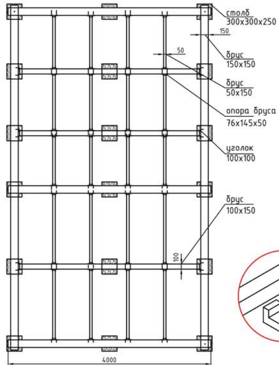
Пример схемы фундамента на столбах:
