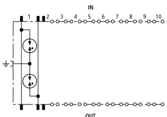
Принципиальная схема DPL 10 G3 110 FSD
