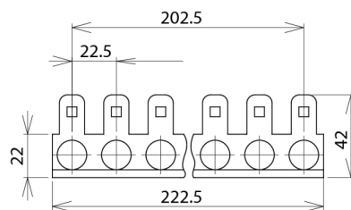
Размерный эскиз MB2 10 LSA
