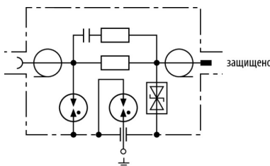
Принципиальная схема UGKF BNC
