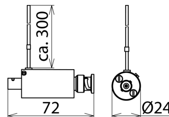
Размерный эскиз UGKF BNC
