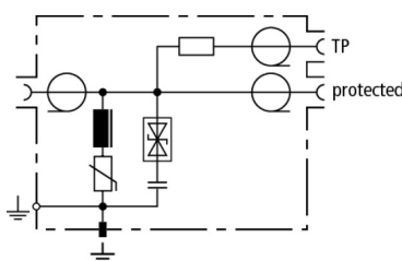
Принципиальная схема DGA FF TV
