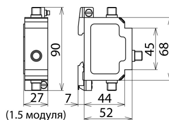
Размерный эскиз DGA FF TV
