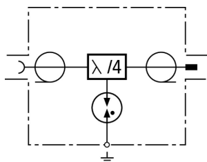
Принципиальная схема DGA LG 7 16 MFA
