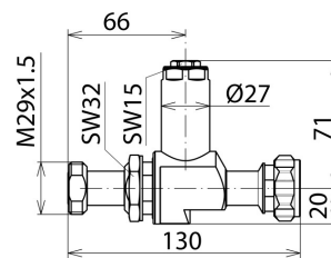
Размерный эскиз DGA LG 7 16 MFA
