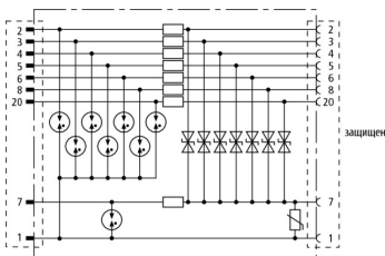
Принципиальная схема USD 25 V24
