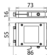
Размерный эскиз USD 25 V24
