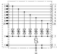
Принципиальная схема FS 25E HS 12
