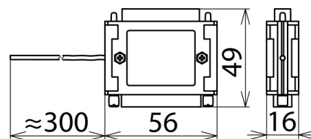
Размерный эскиз FS 25E HS 12
